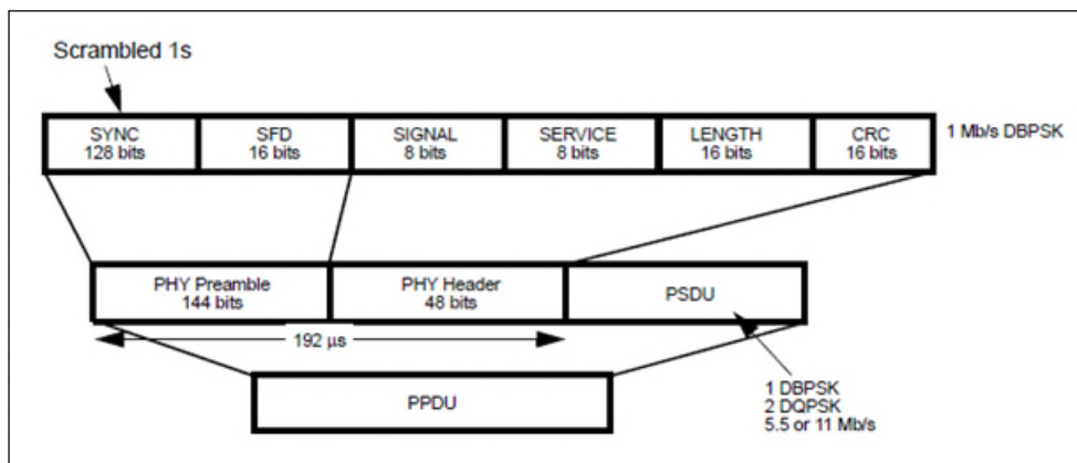
Long PDU Format, IEEE STD 802.11-2016 at Fig. 16-1.
