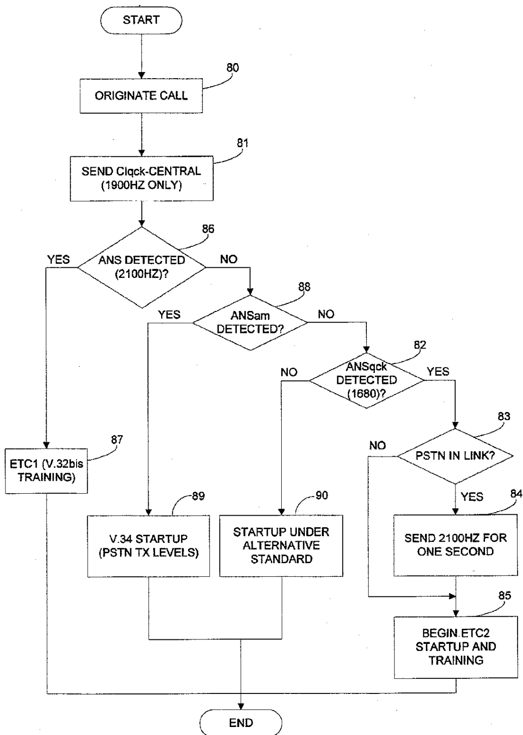
Calling Modem -- Central Site FIG. 6
